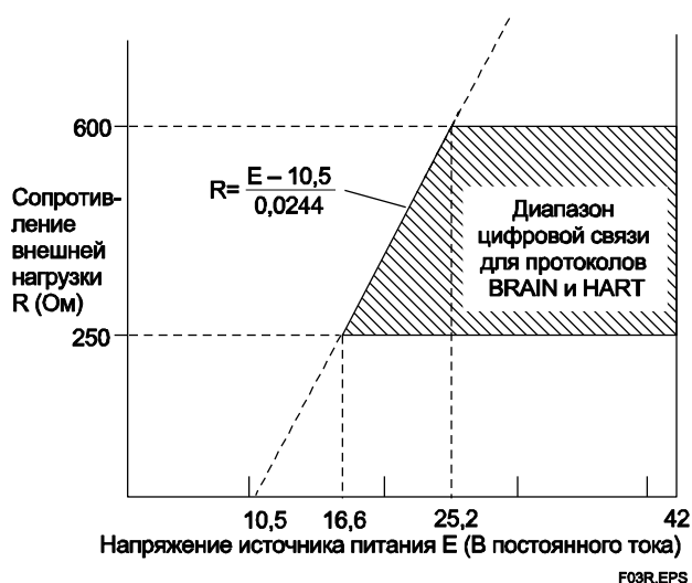
Рис. 2. Связь напряжения питания и сопротивления внешней нагрузки
